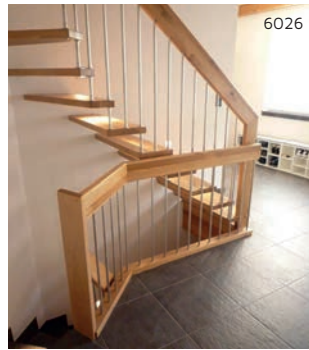
6026 Freistehendes Brüstungsgeländer
