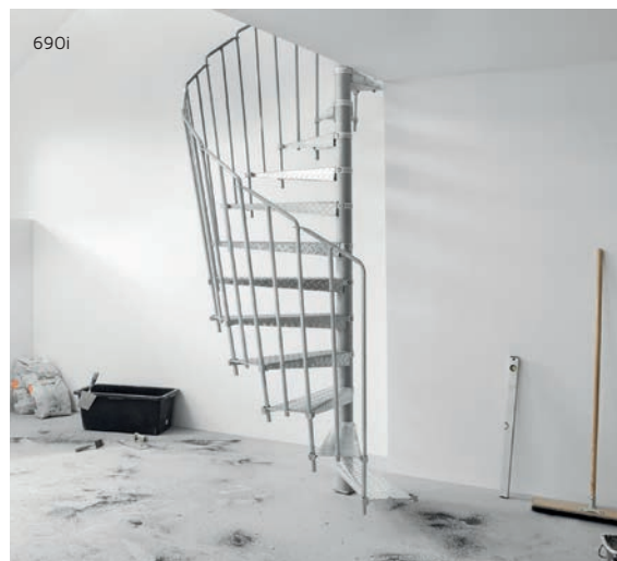
Die Bautreppe aus Stahl ist vom TÜV Süd mit der Nr. Z1 16 03 93563 002 zertifiziert.
