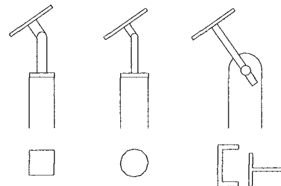
Handlaufvarianten
